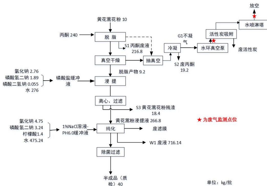
图 7.1.1-1 有组织废气监测点位示意图
